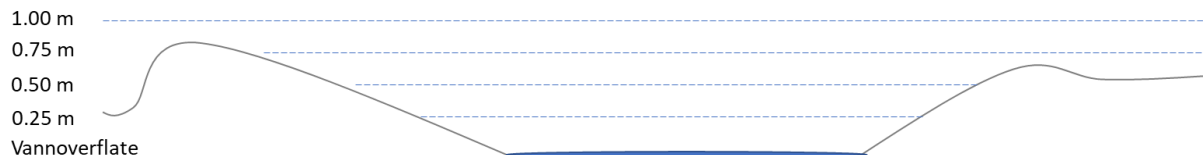
Figur 21: Tverrsnitt av vannmettet område og områder som kan bli vannmettet ved stigende vannmengde. Dersom terrenget består av løsmasser vil vann også trenge inn i grunnen.
